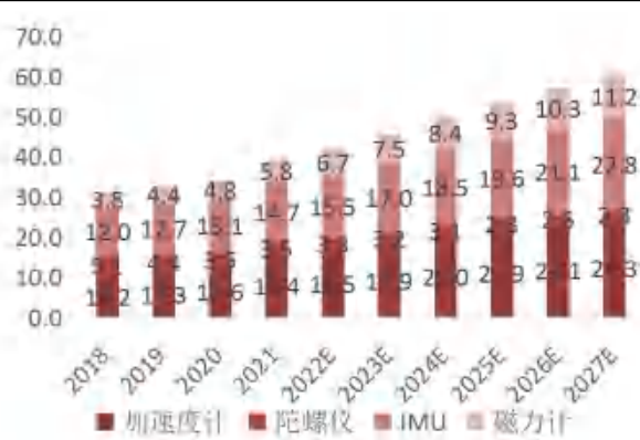
图 23：全球 MEMS 惯性传感器市场结构（亿颗）
