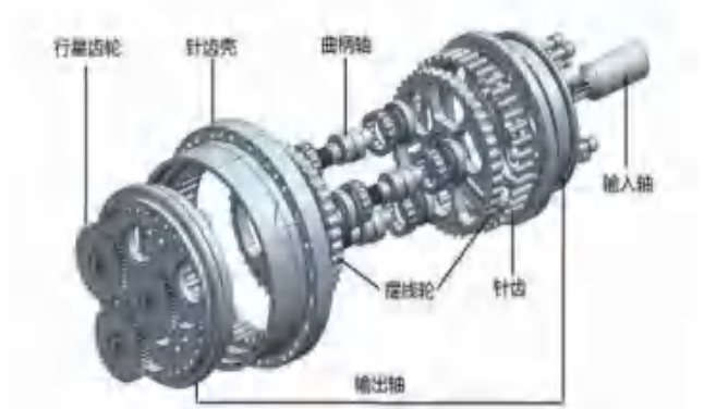
图 27：RV 减速器结构图
