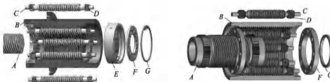
图 34：标准式 VS 反向式行星滚柱丝杠
