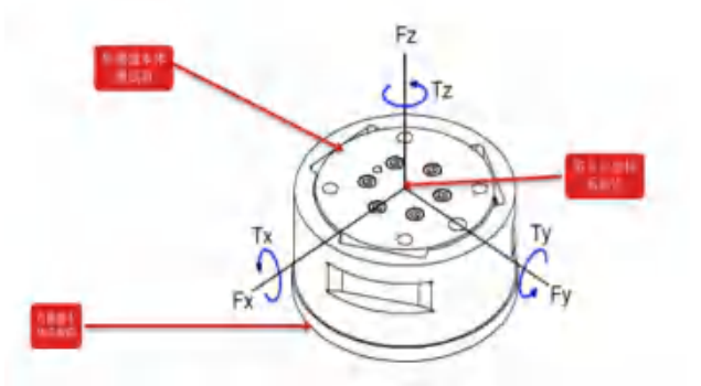
图 15：六维力/力矩传感器
